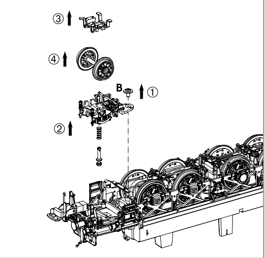
Vorläuferdemontage / Precursor disassembly Démontage du précurseur / Forerunner demontage
