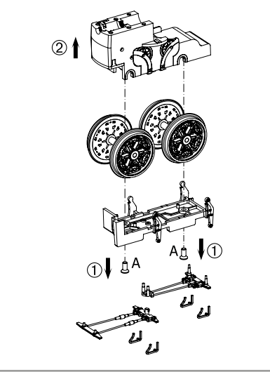
Radsatzdemontage / Wheelset disassembly Démontage des roues / Demontage wielstel
