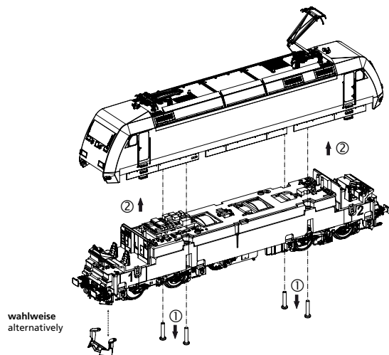
Gehäusedemontage: Body disassembly
