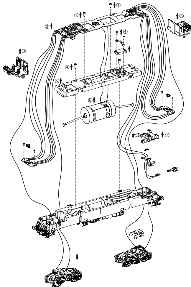
Leiterplatte + Motor ausbauen: Remove main board+motor
