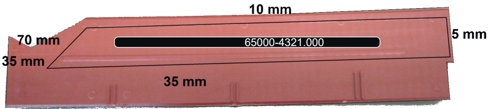
65000-0823.050 + 1x 65000-4321.000
